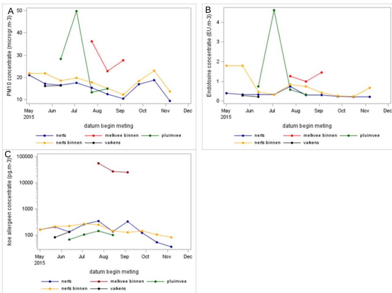
Figuur 2. Verloop over de tijd van concentraties PM10 (a), endotoxine (b) en koe-allergeen (c) voor de meetlocaties bij nertsenhouders (binnen en buiten), pluimveehouderij (buiten), melkveehouderij (binnen) en varkenshouderij (buiten).
